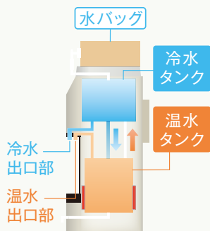
高温循環システム イメージ図
